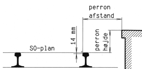
Figur 10.1-1 Illustration af måling af perronafstand og perronhøjde for spor uden overhøjde.
