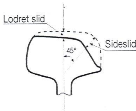
figur 13.2.1-1 Måling af skinnerlid
